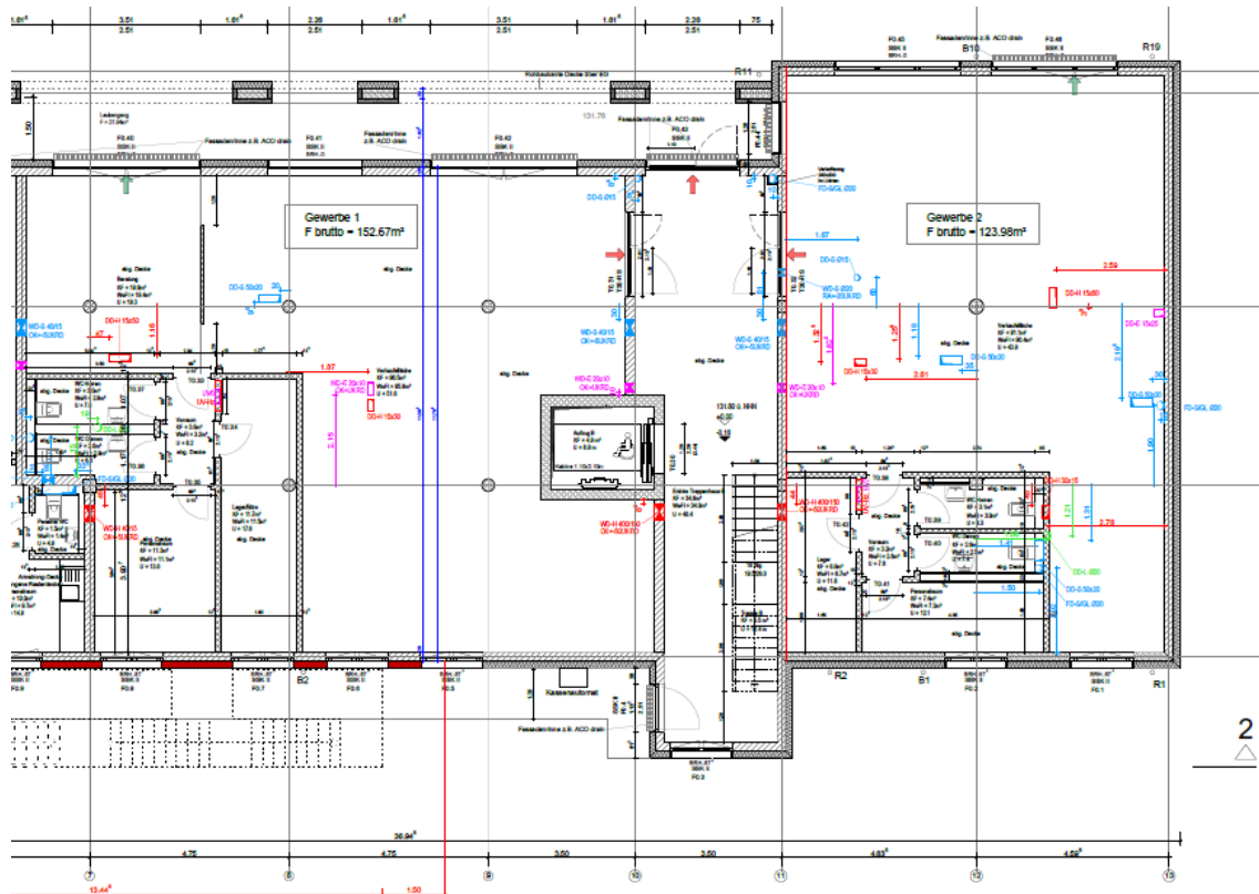
Grundrisse Gewerbefläche 1 und 2
